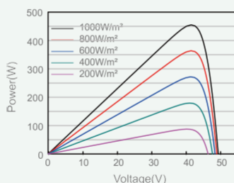
Power-Voltage Curve(SP455M-72H)
